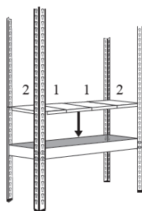
Рис.5а Укладка металлического настила
