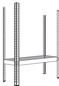
Рис.6а Вид стеллажа без настила под шины
